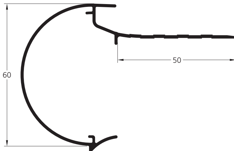
Numéro d'article 147635 (échelle 1:1)
