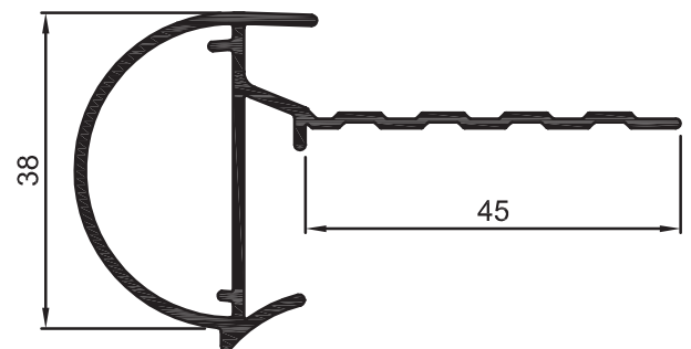
Numéro d'article 147628 (échelle 1:1)
