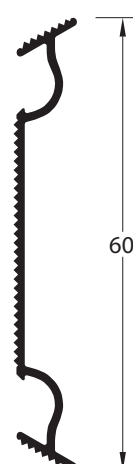
Numéro d'article 151599 (échelle 1:1)
