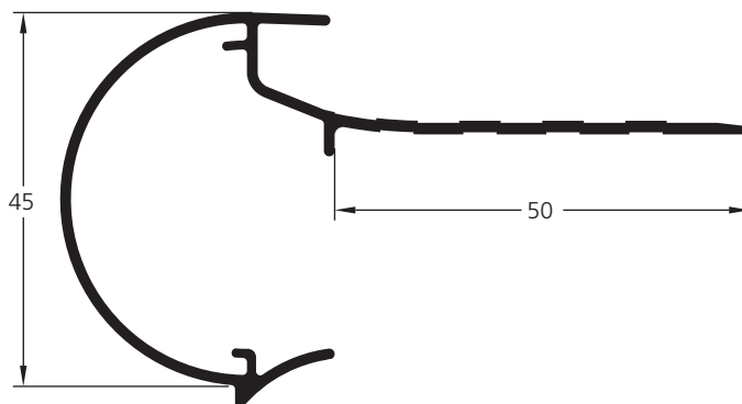
Numéro d'article 147632 (échelle 1:1)
