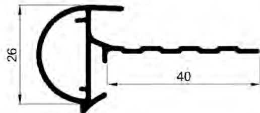
Numéro d'article 147626 (échelle 1:1)
